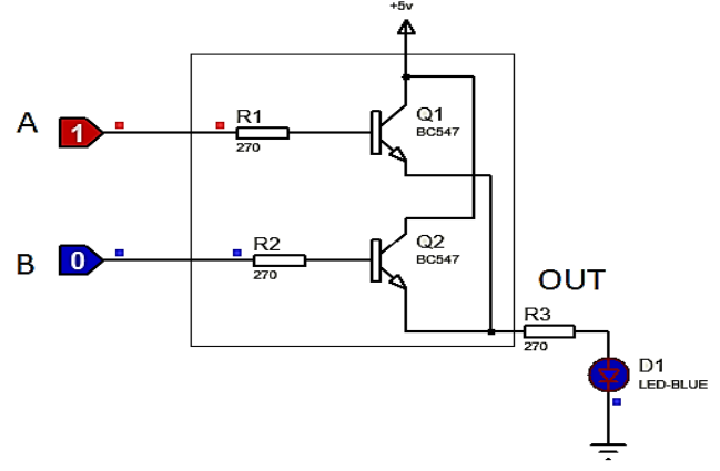
Fig.: OR gate
